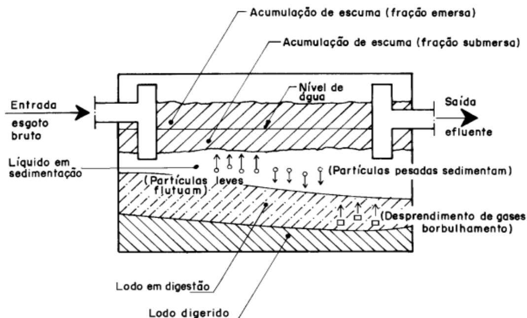
Figura 7 - Esquema de um tanque séptico.
