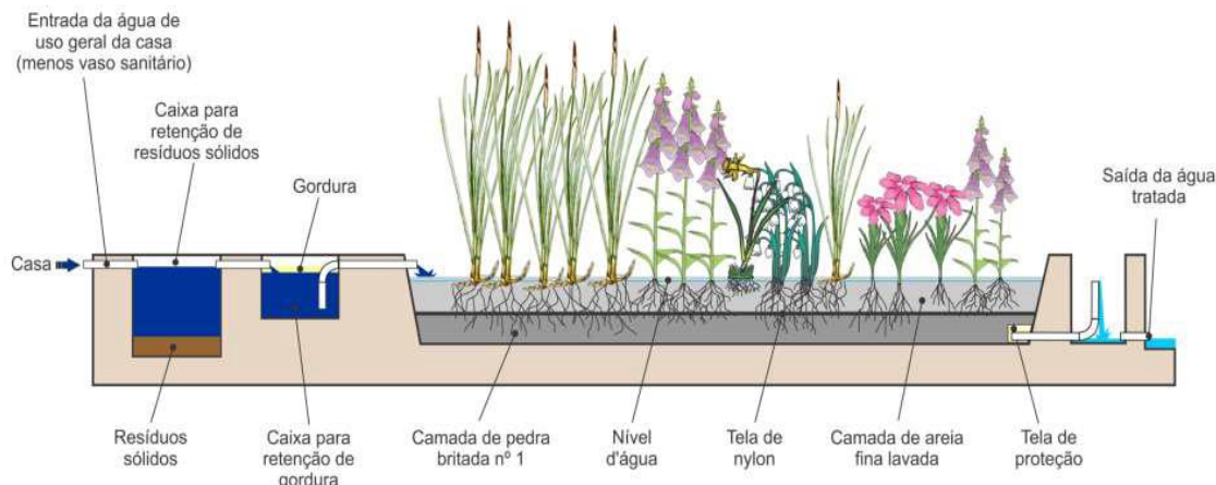
Figura 6 - Esquema em Corte de um Jardim Filtrante.
