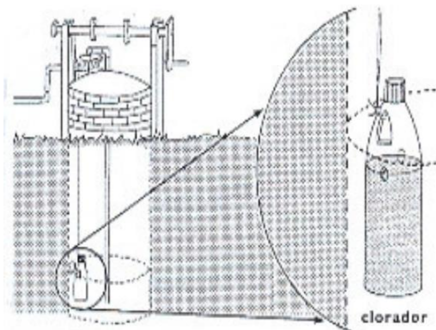
Figura 3 - Garrafa Dosadora de Cloro.
