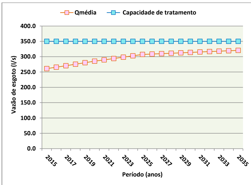
Gráfico 5 - Capacidade de Tratamento x Geração de Esgoto.
