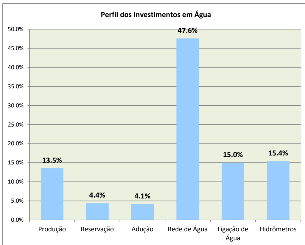
Gráfico 8 - Perfil dos Investimentos no Sistema de Abastecimento de Água.
