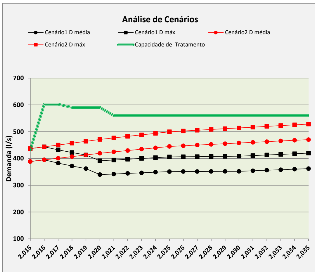
Gráfico 4 - Análise dos Cenários de Produção.
