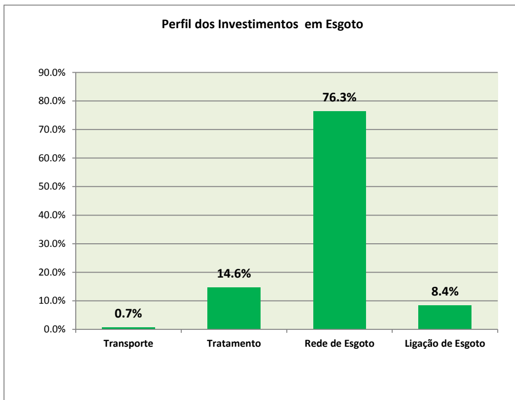
Gráfico 9 - Perfil dos Investimentos no Sistema de Esgotamento Sanitário.
