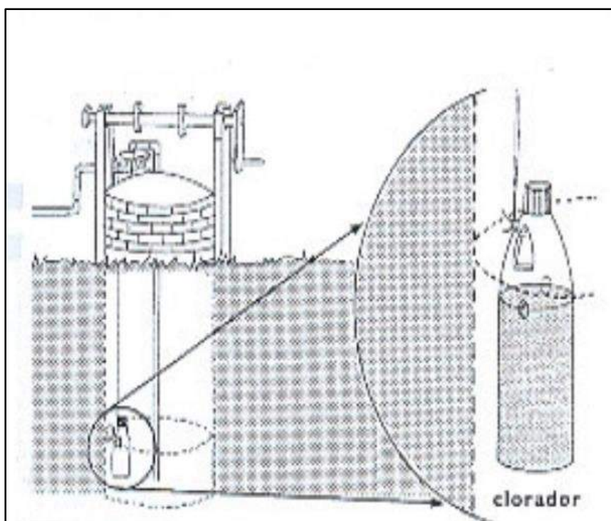
Figura 4 - Garrafa Dosadora de Cloro.
