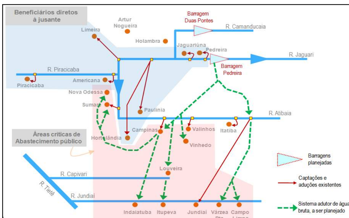
Figura 1 - Esquema do Sistema Adutor Regional.
