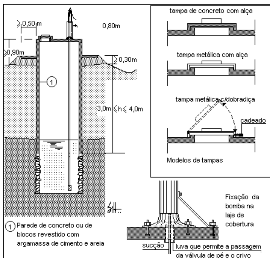
Figura 3 - Proteção de Poços Rasos.
