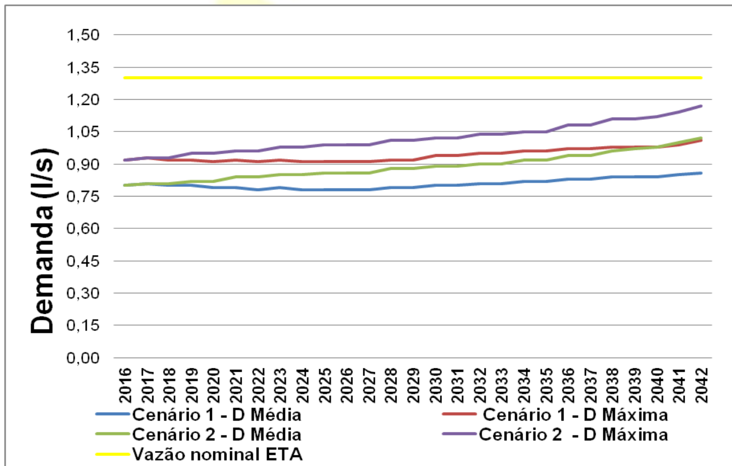
Gráfico 4 - Análise dos cenários de produção - Princesa da Colina
