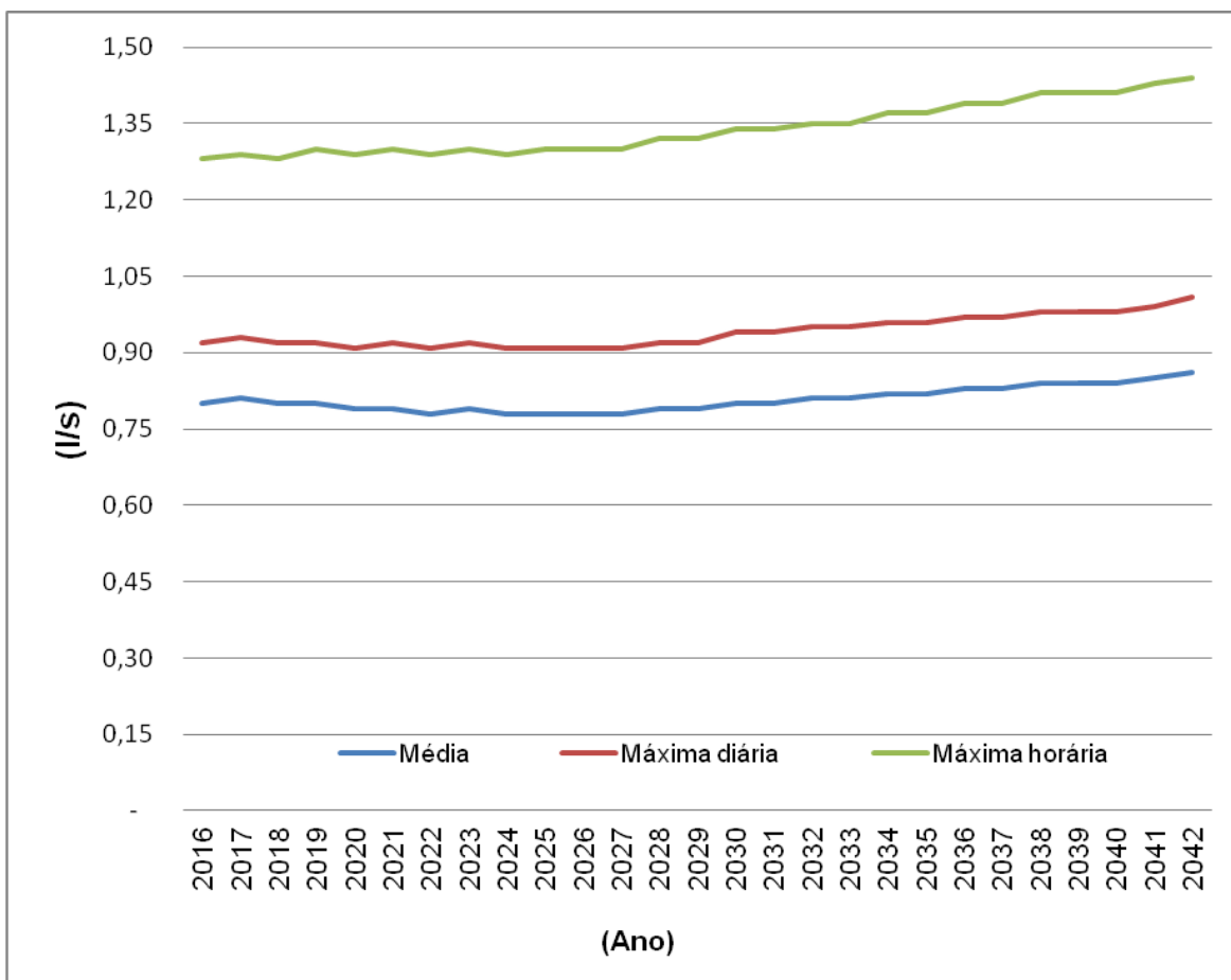
Gráfico 2 - Análise das demandas – Princesa da Colina
