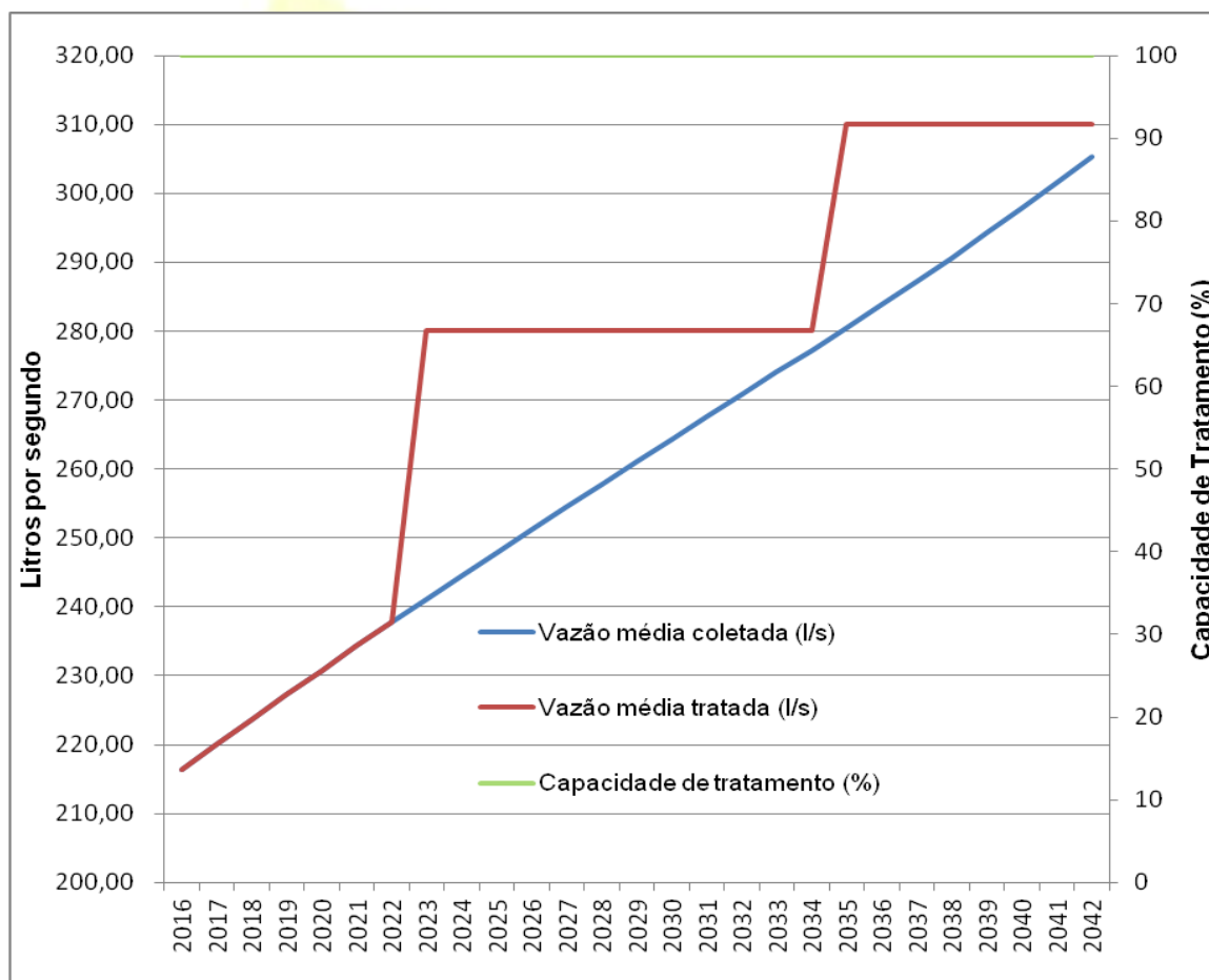
Gráfico 5 - Projeção das vazões de tratamento e coleta de esgoto - Sede
