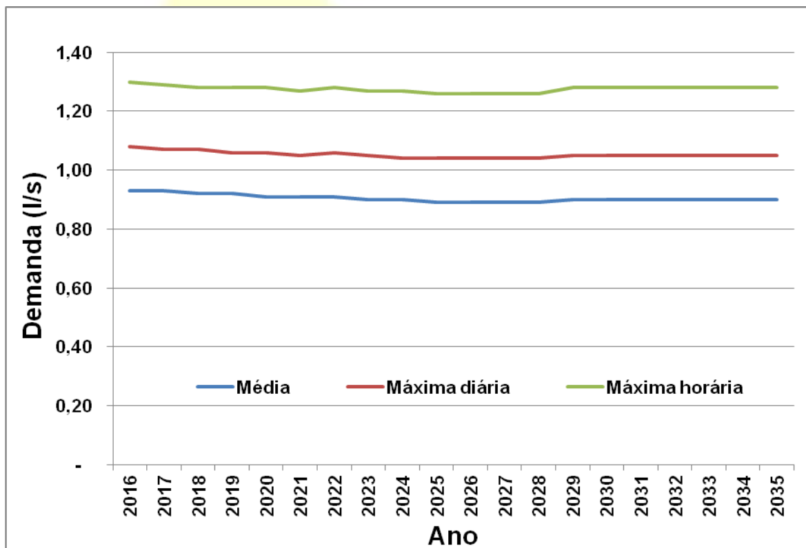
Gráfico 3 - Análise das demandas do bairro Ferreira
