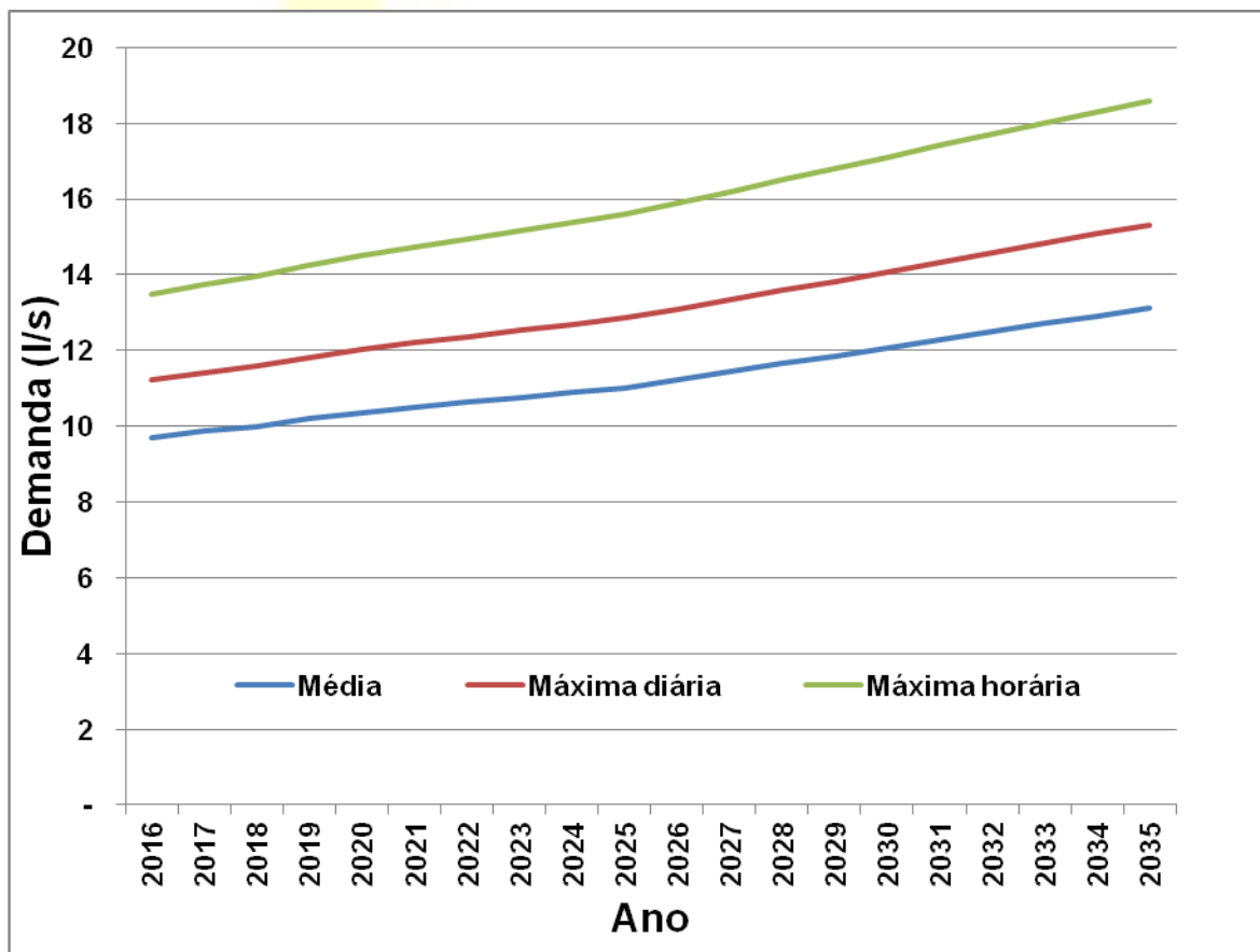
Gráfico 1 - Análise das demandas - Sede
