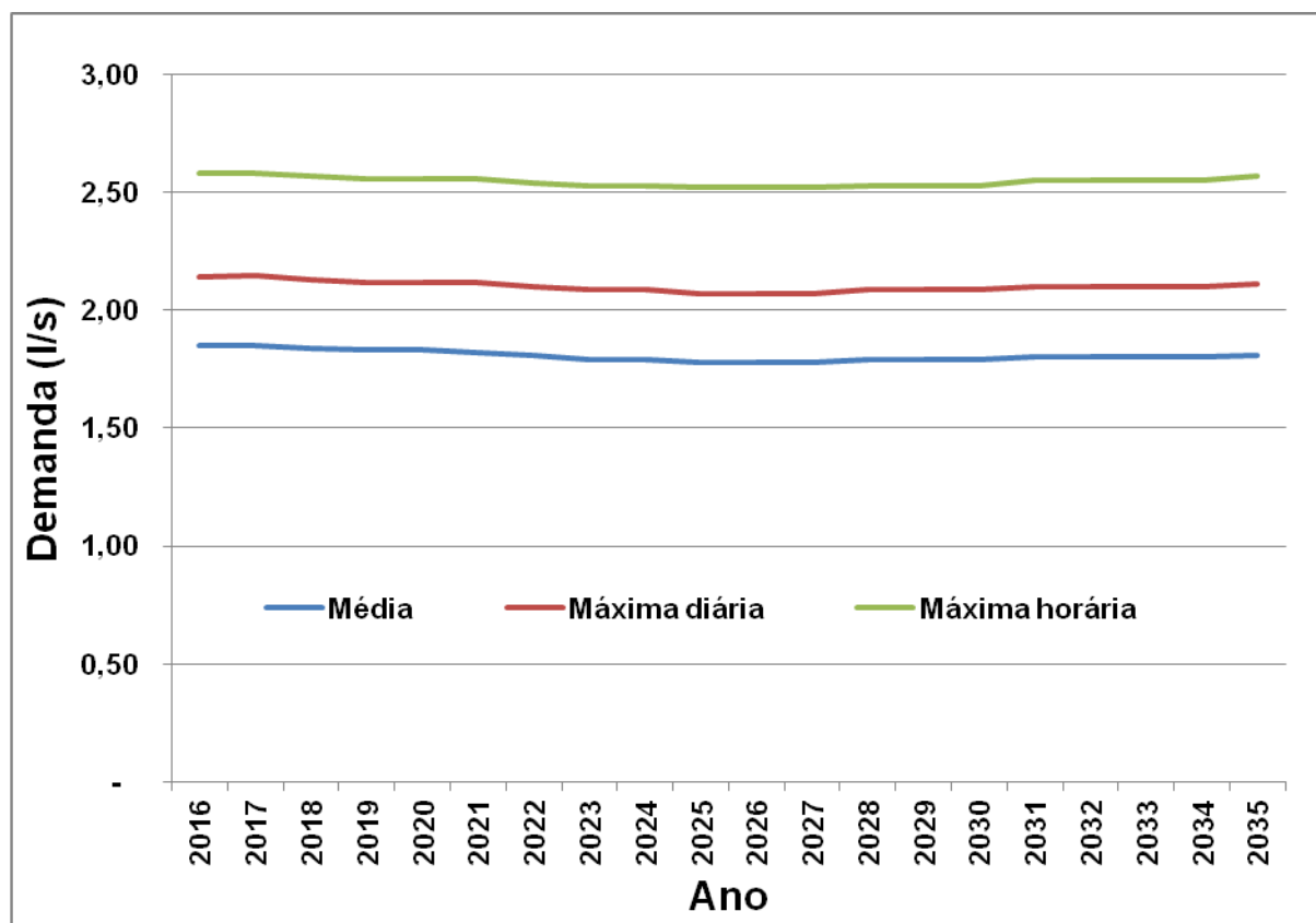
Gráfico 5 - Análise das demandas do bairro Tropical Flores
