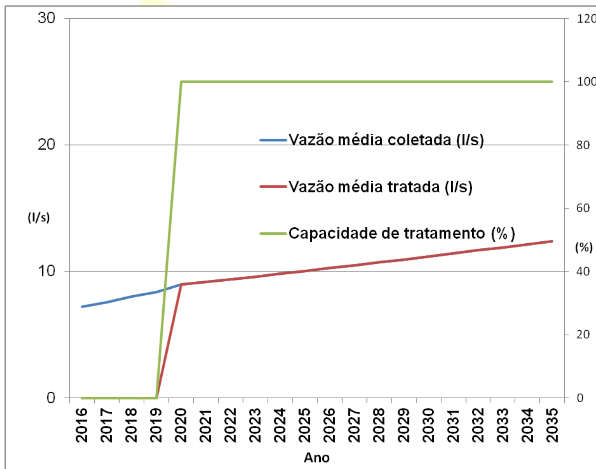
Gráfico 7 - Evolução da vazão média e da capacidade de tratamento - Sede
