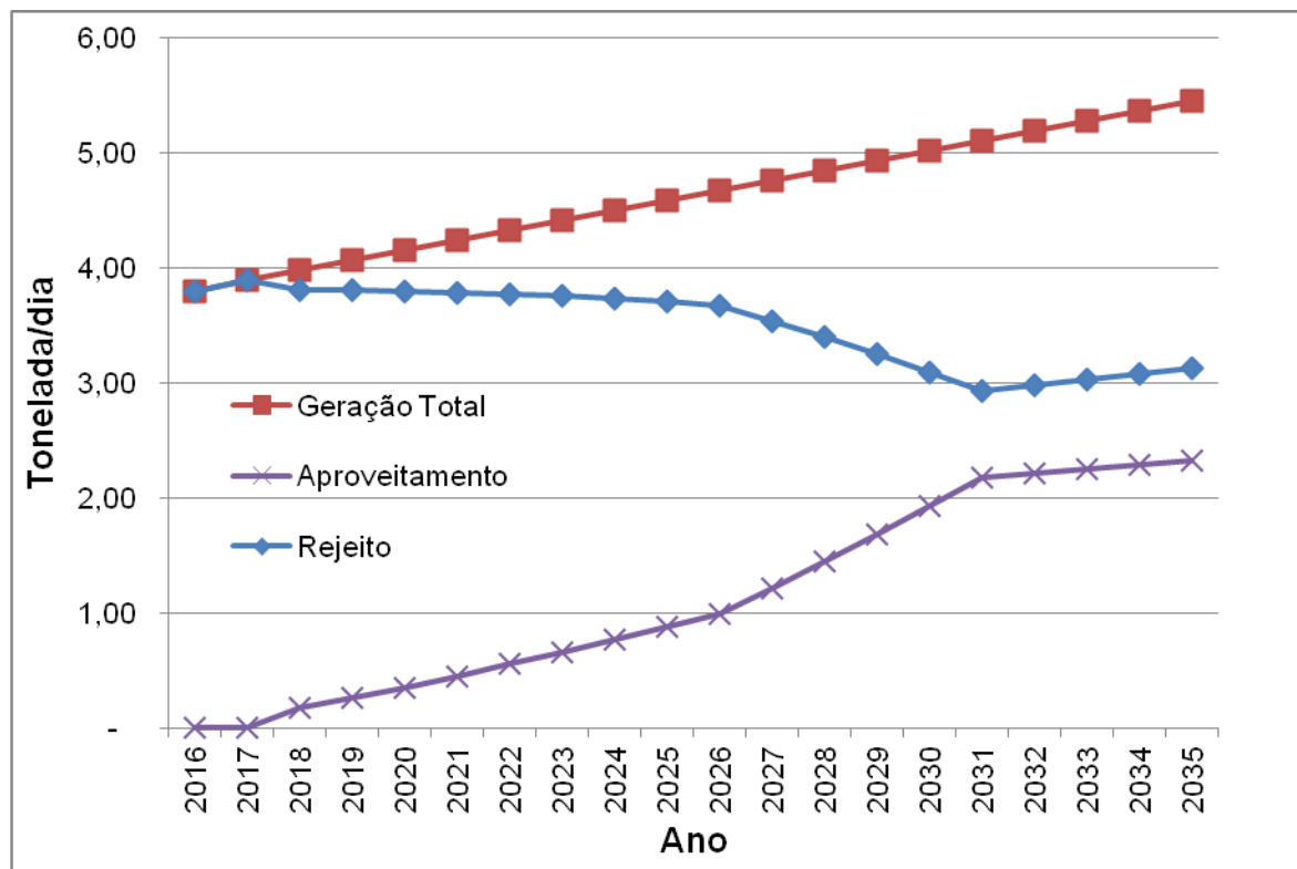
Gráfico 17 - Balanço entre produção e aproveitamento de resíduos sólidos
