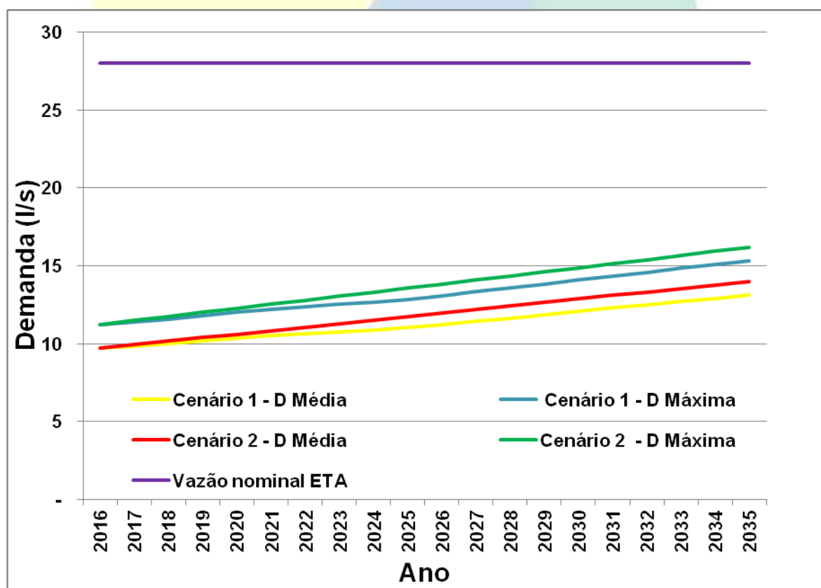
Gráfico 6 - Análise dos cenários de produção - Sede
