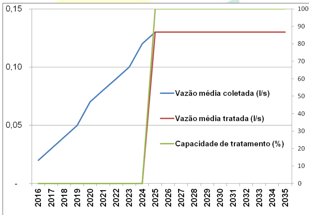
Gráfico 8 - Evolução da vazão média e da capacidade de tratamento – bairro Sertão Grande
