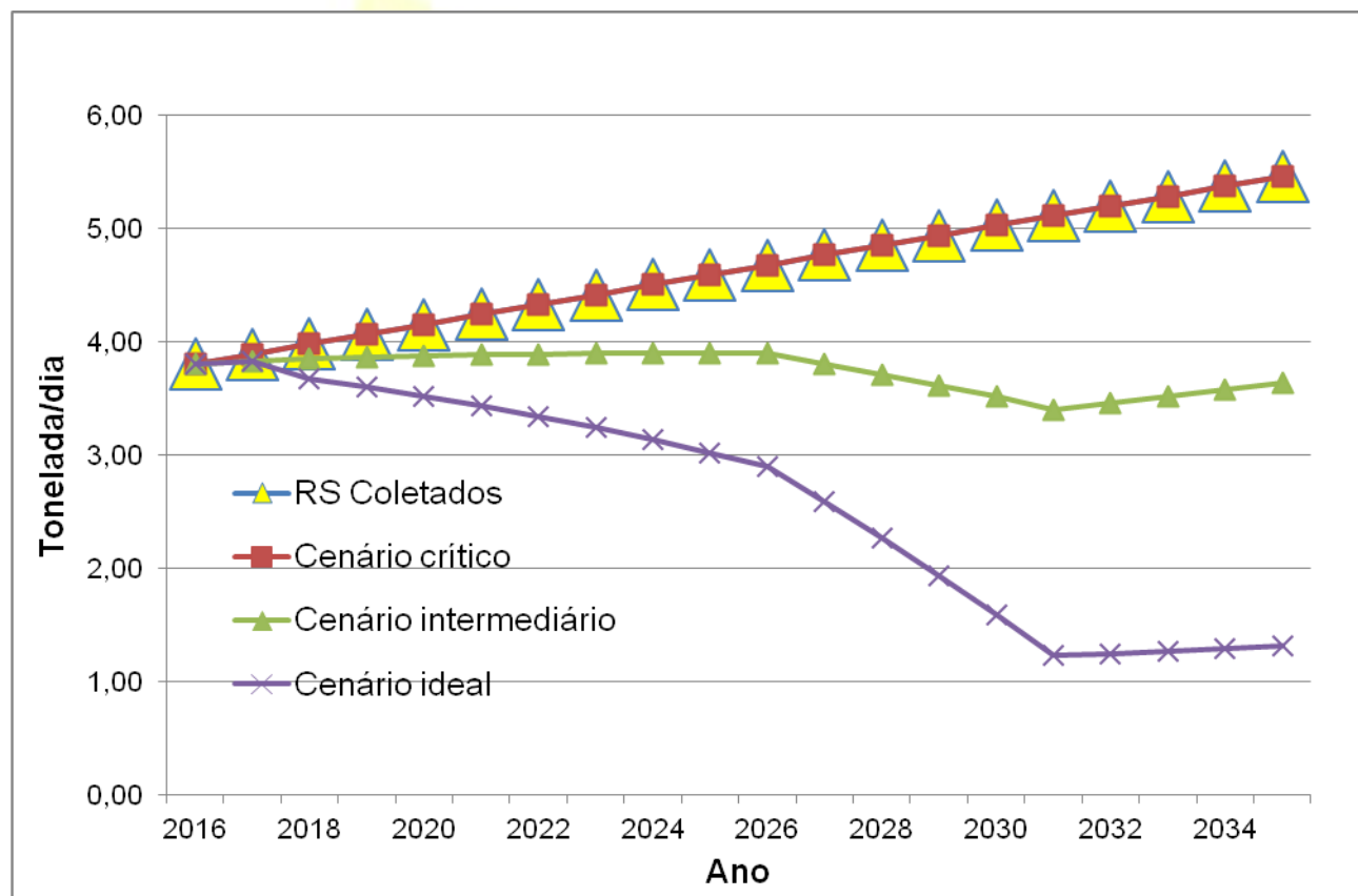
Gráfico 18 - Balanço entre produção e aproveitamento
