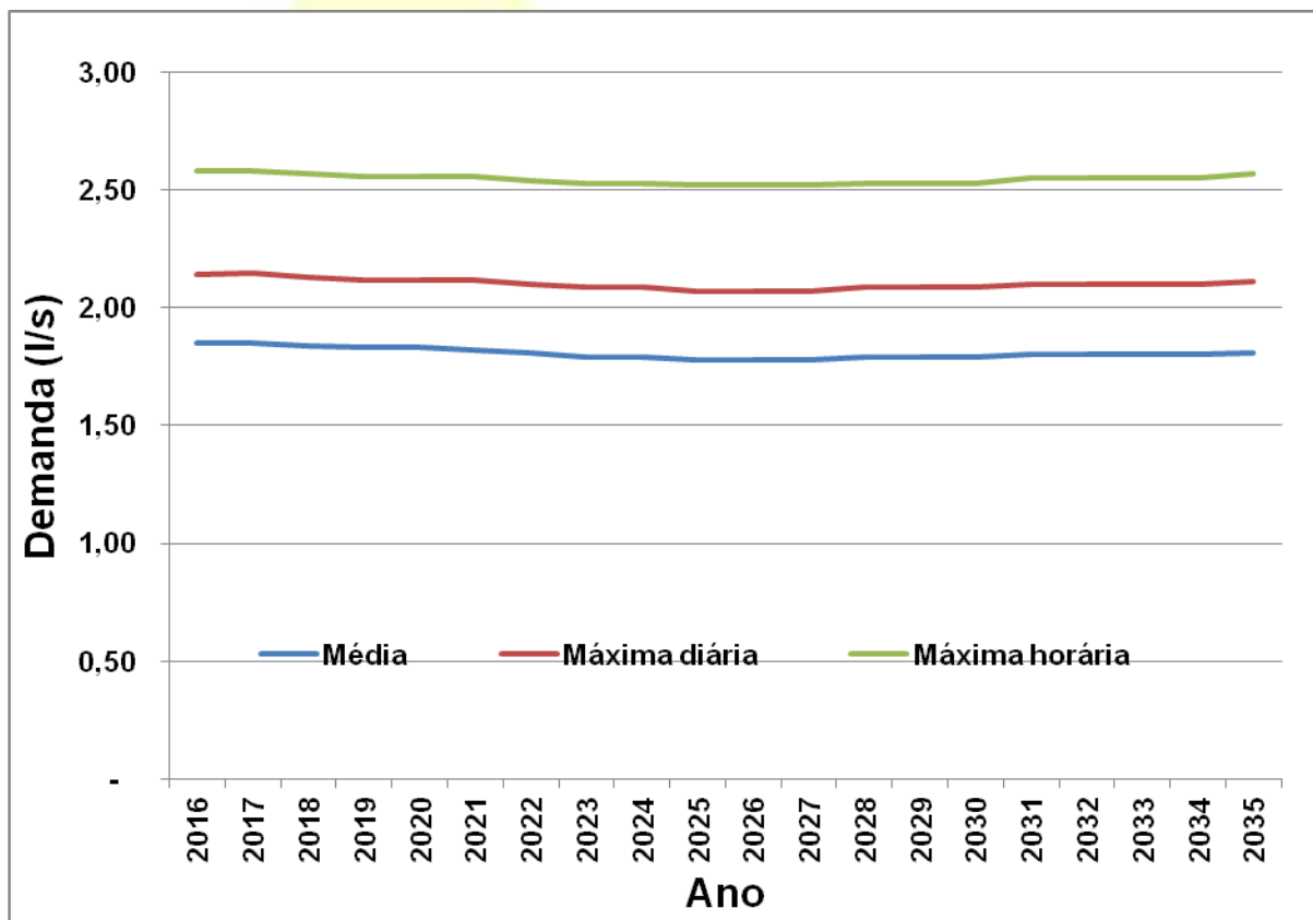
Gráfico 4 - Análise das demandas do bairro Areias
