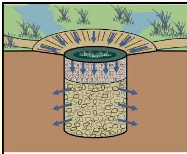
Figura 30 - Dispositivo de controle de escoamento – Poço de infiltração
