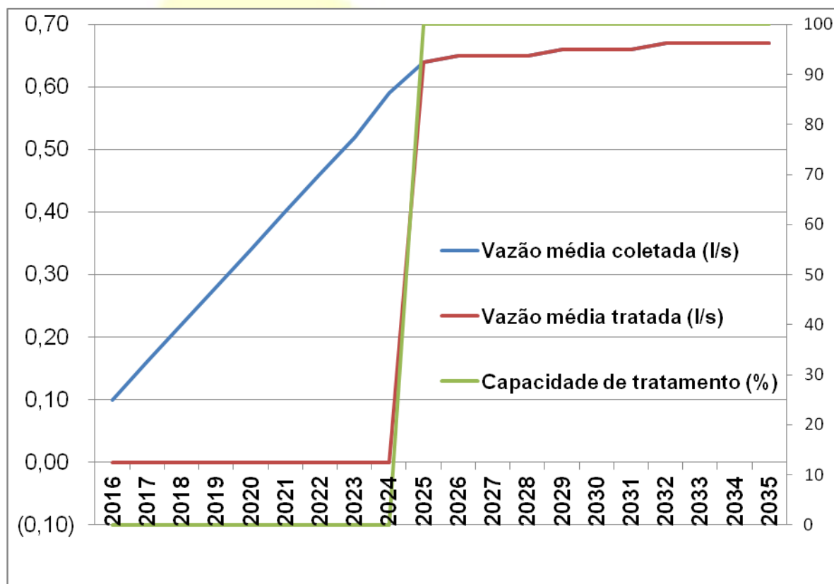
Gráfico 9 - Evolução da vazão média e da capacidade de tratamento - bairro Ferreira
