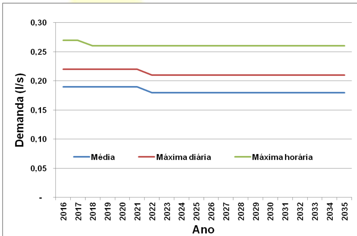
Gráfico 2 - Análise das demandas do bairro Sertão Grande
