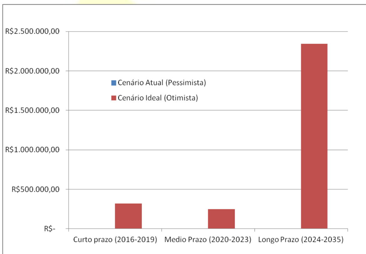
Gráfico 24 - Programa de implantação de sistema de monitoramento, previsão e alerta de enchentes
