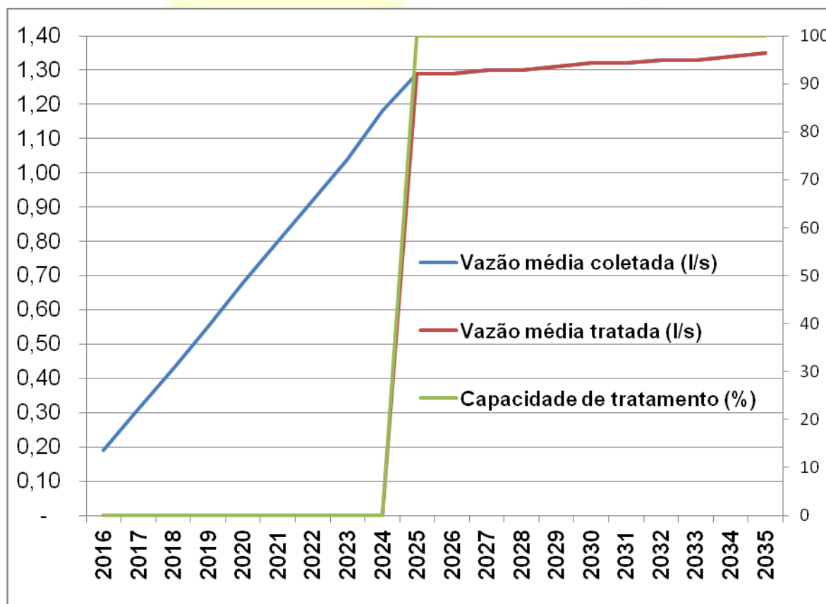
Gráfico 10 - Evolução da vazão média e da capacidade de tratamento – bairro Areias
