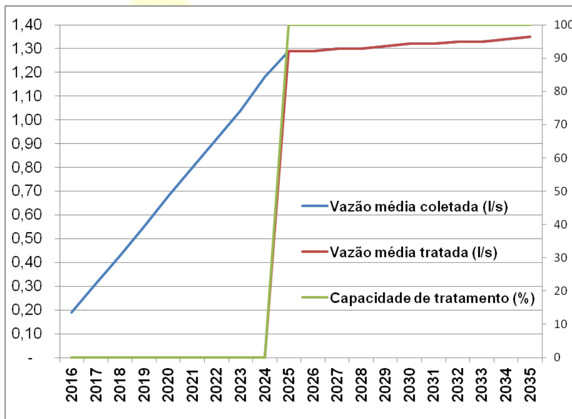
Gráfico 11 - Evolução da vazão média e da capacidade de tratamento – bairro Tropical Flores
