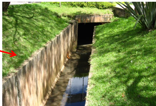
Figura 18 - Vista da canalização do Córrego Divinéia e aduela da travessia sob a Rodovia Fernão Dias. Ampliação da canalização e aduelas existentes;
