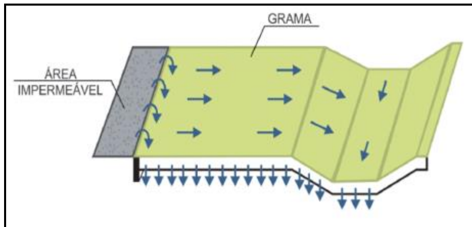
Figura 19 - Dispositivo de controle de escoamento – Faixas Gramadas.
