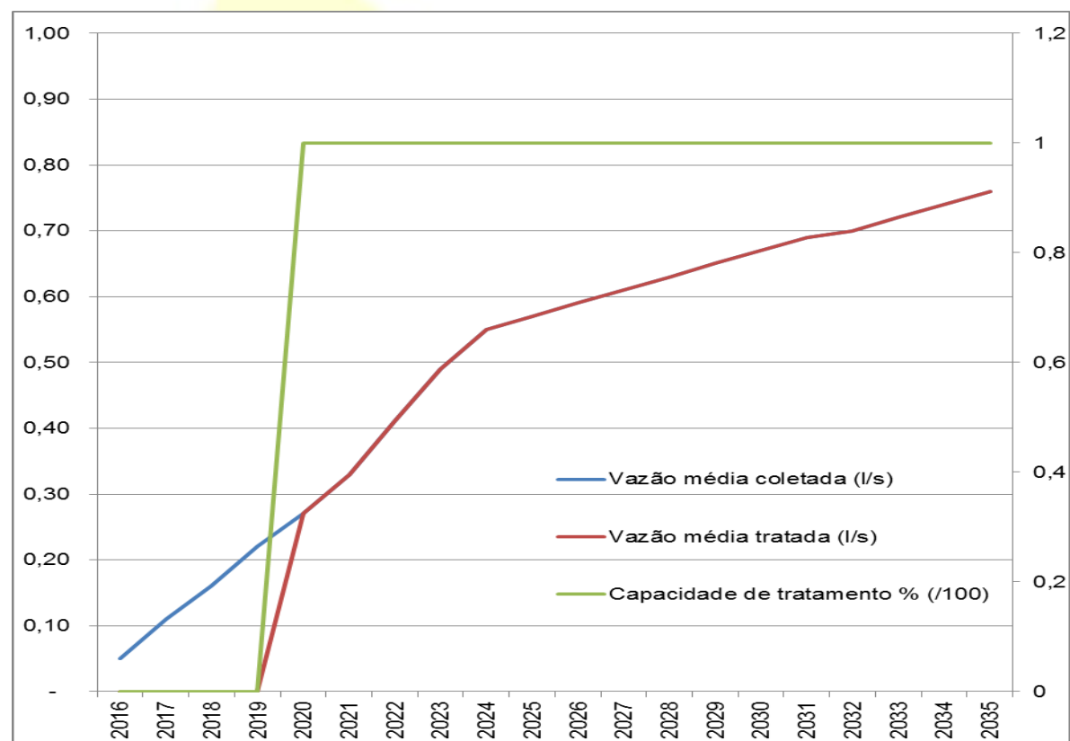
Gráfico - 9 Projeção das vazões de tratamento de esgoto - São Mateus de Minas
