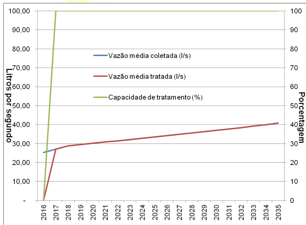
Gráfico - 7 Projeção das vazões de tratamento de esgoto - Sede
